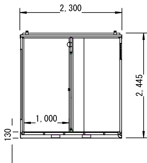
右側面図
