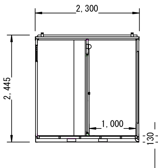
左側面図
