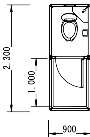
平面図
