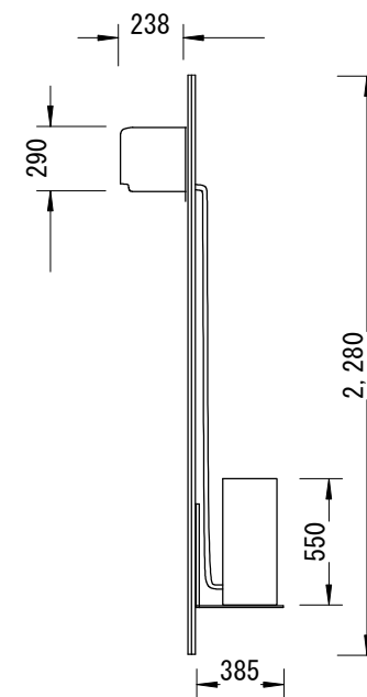
右側面図
