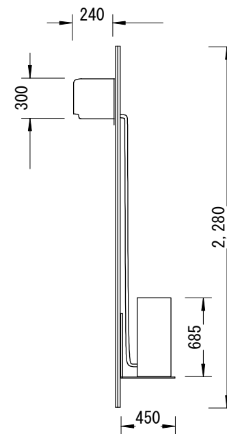
右側面図
