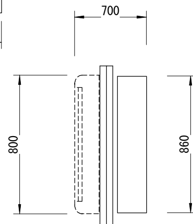
平面図
