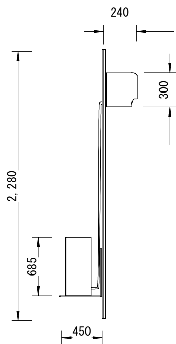
左側面図
