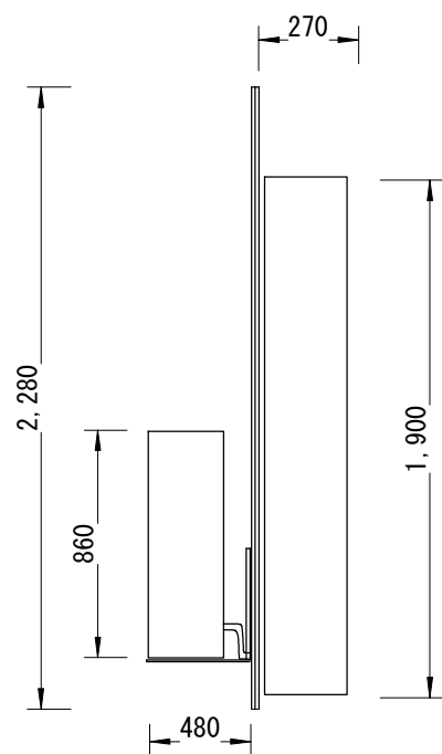
左側面図
