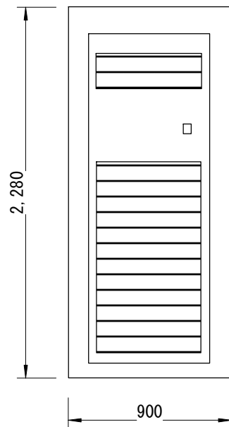
正面図
