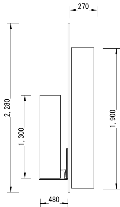
左側面図
