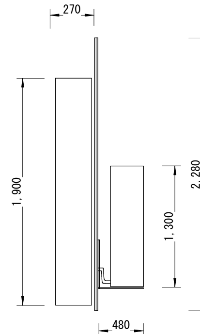
右側面図
