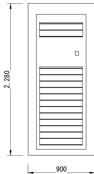
正面図
