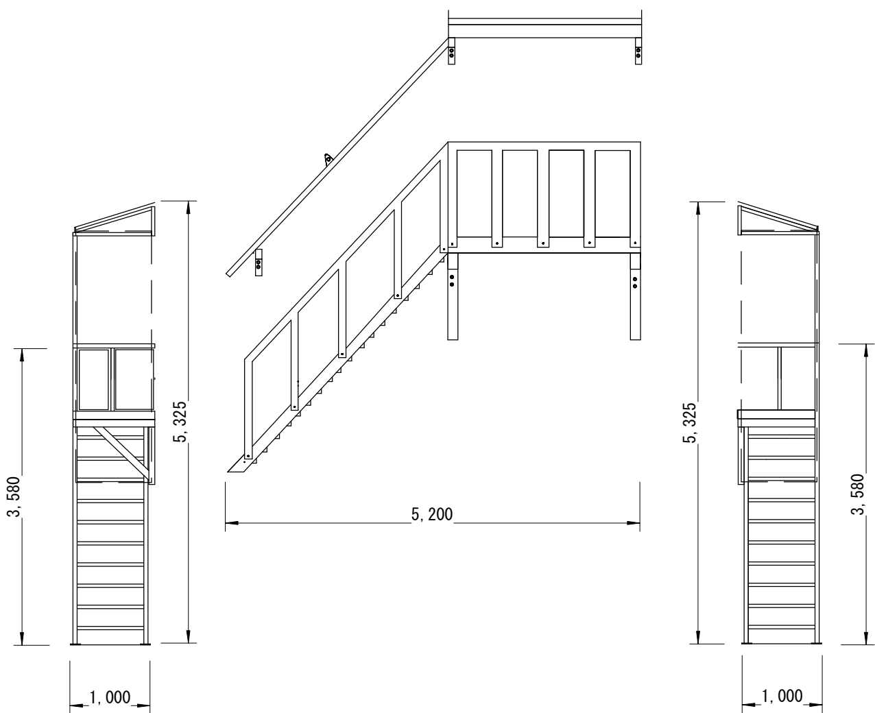
正面図
