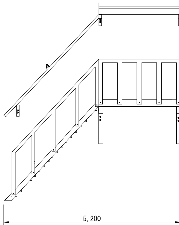
正面図
