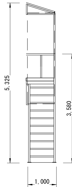
左側面図
