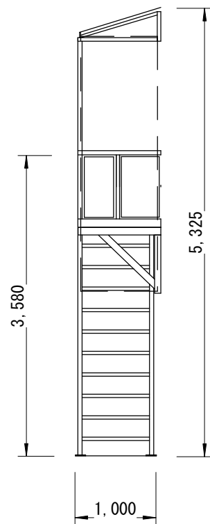
右側面図
