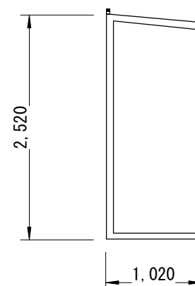
右側面図
