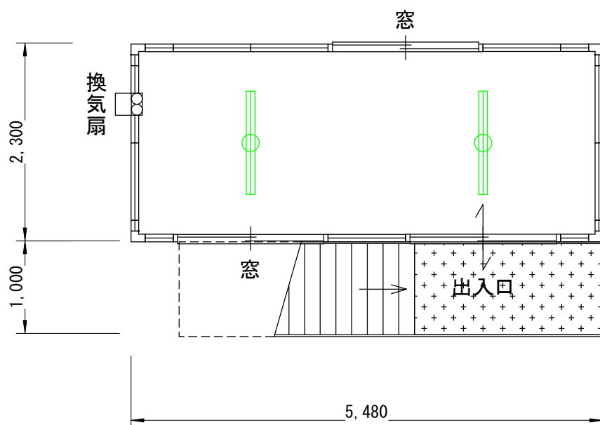
2階平面図
