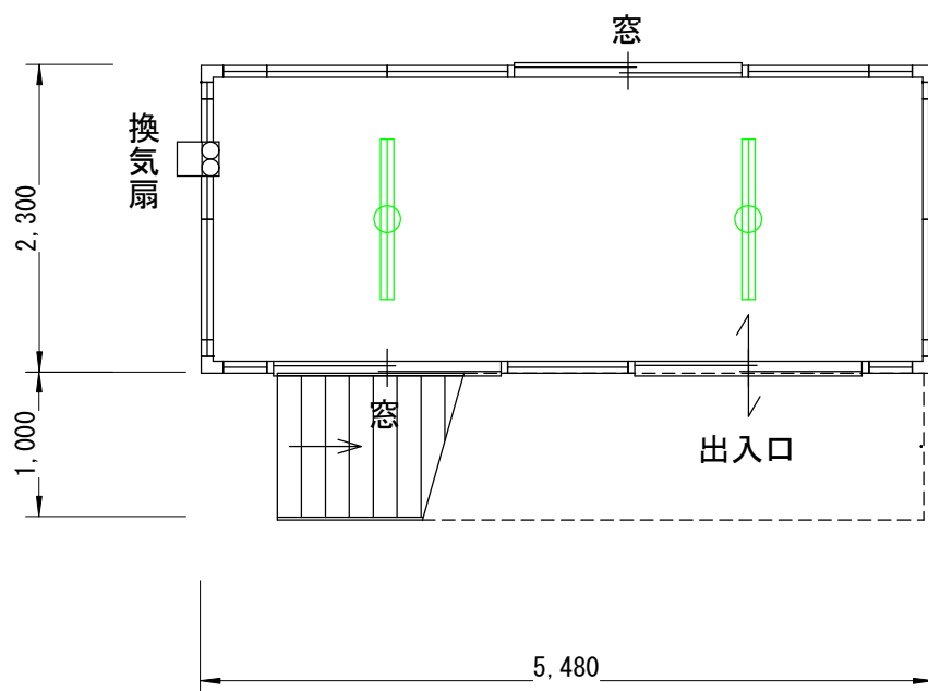
1階平面図
