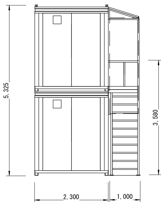
左側面図
