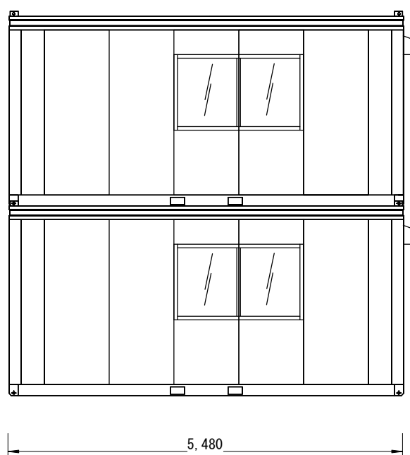
後面図
