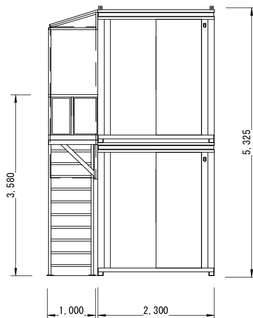
右側面図
