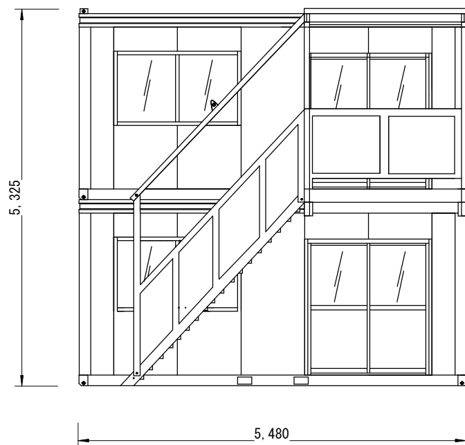
正面図
