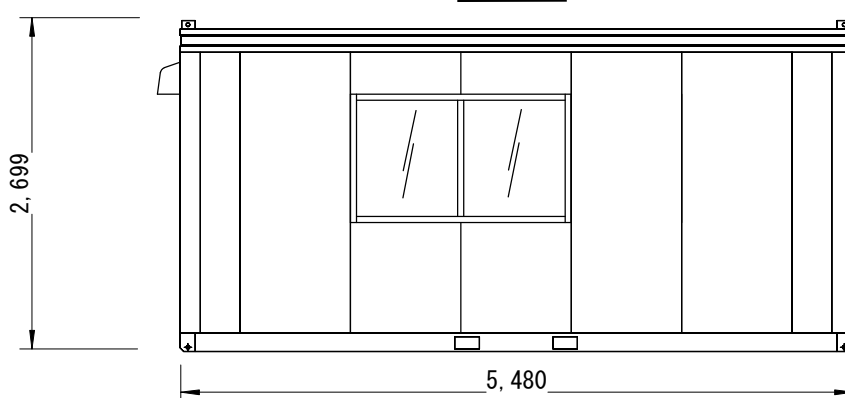
左側面図
