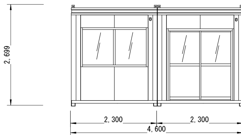
正面図
