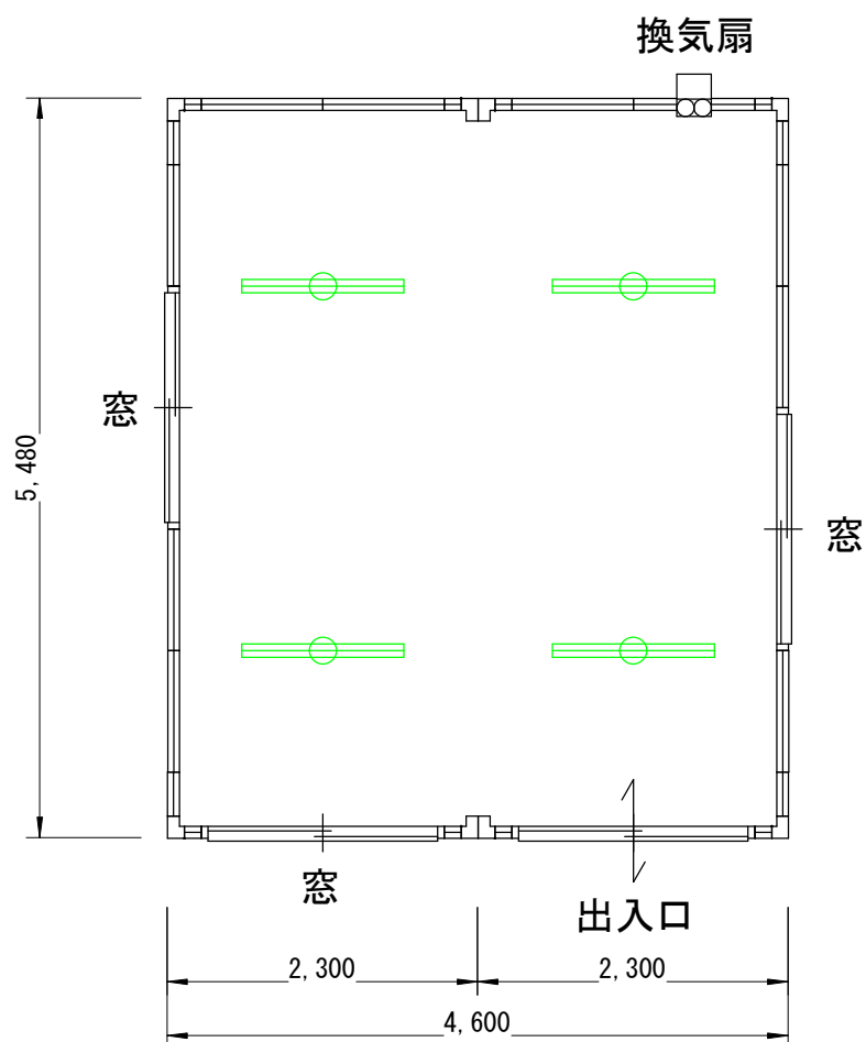
平面図
