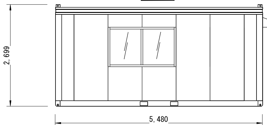
右側面図
