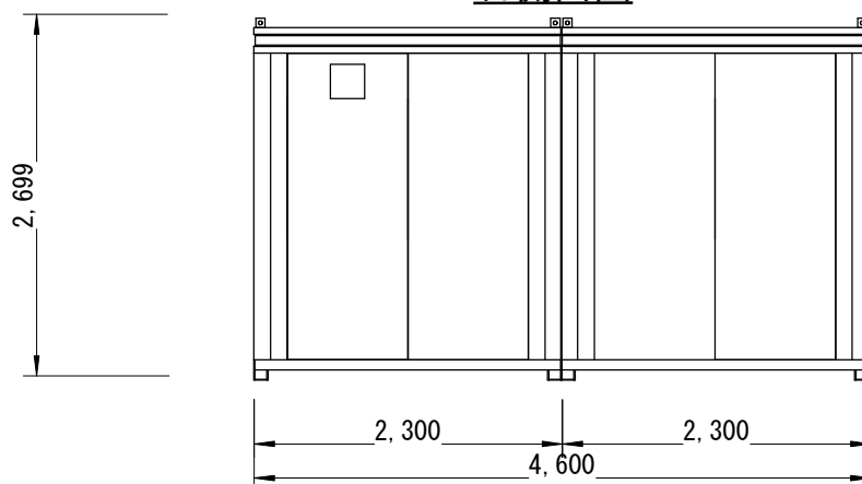
後面図
