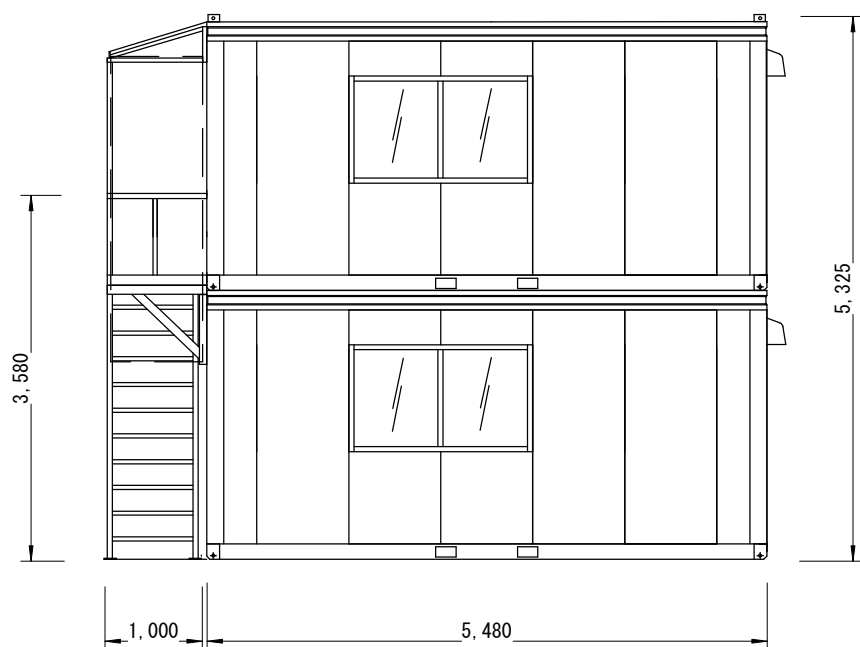
右側面図
