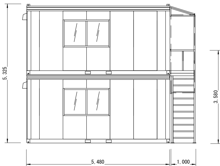
左側面図
