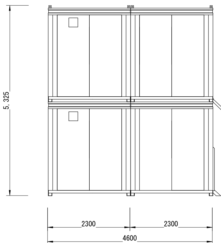
後面図
