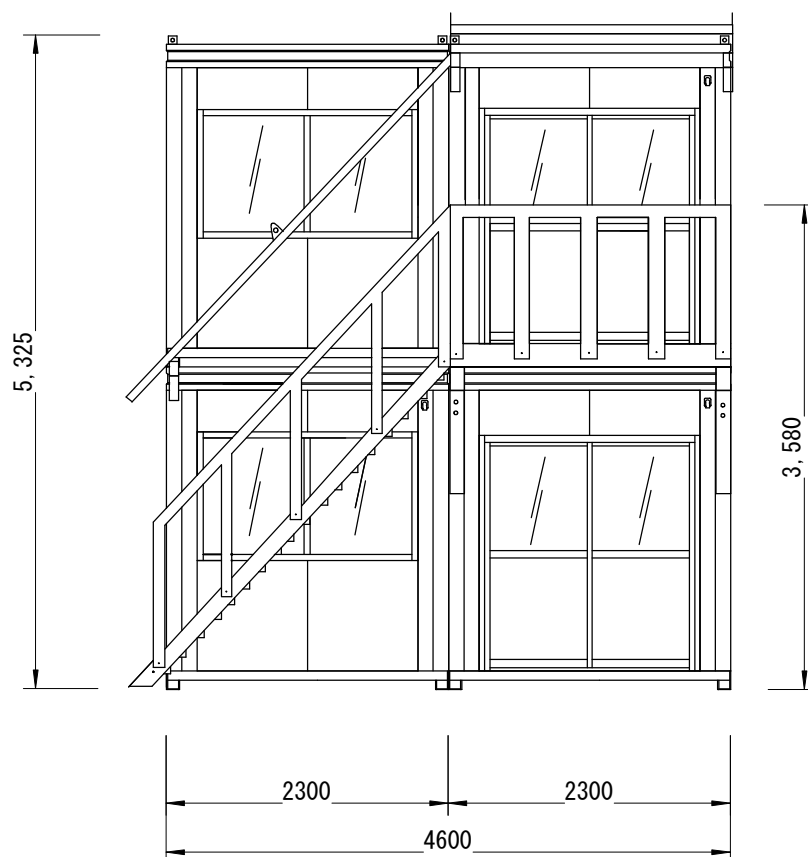
正面図
