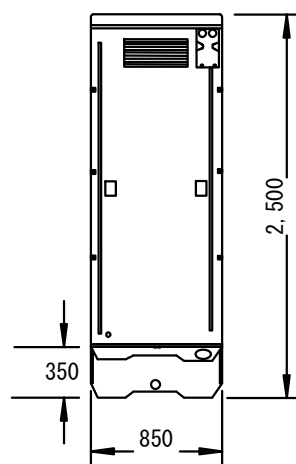
後面図
