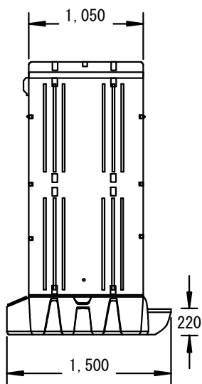
左側面図
