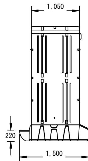
右側面図
