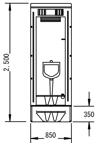
正面図
