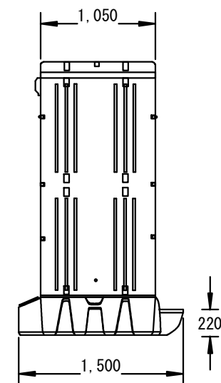
左側面図
