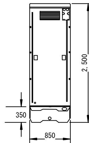
後面図
