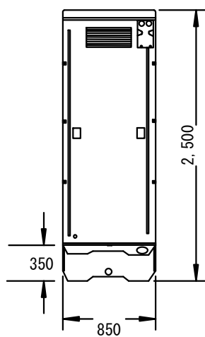
後面図
