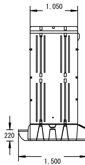
右側面図
