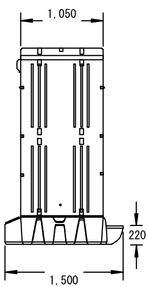
左側面図
